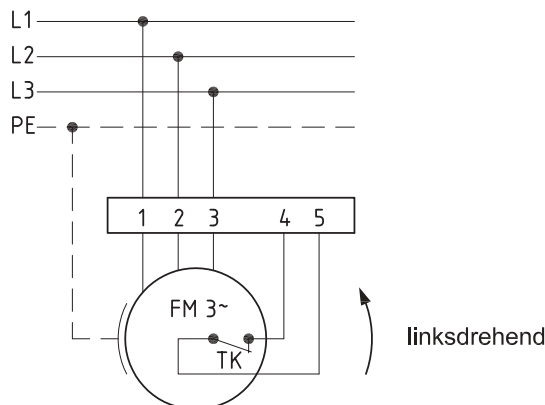
Anschlußplan 0.13-2 I.
